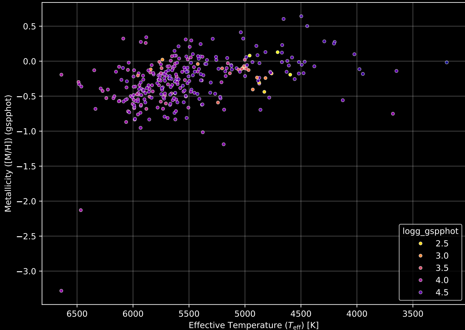
GALAH DR4 Field: [6962] Stellar Population Parameters (n= 309)
